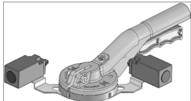
Levier avec deux fins de course SPDT ou inductifs*
