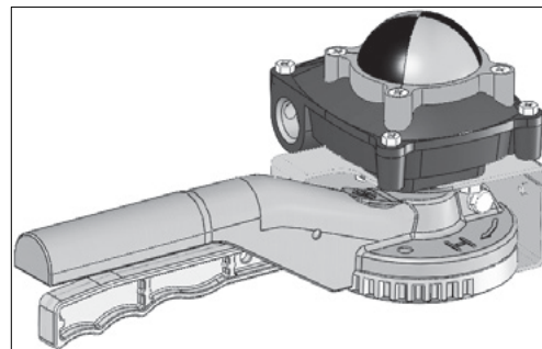
Levier avec deux fins de course SPDT ou inductifs*
